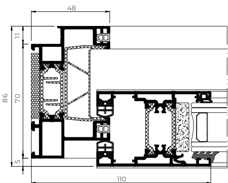
SIDE JAMB
