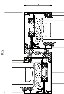
INTERLOCK
